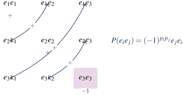
Şekil 9.2 Süper permutasyon P , V \otimes V bazı üzerinde bir takas: köşegen-dışı çiftler işaretsiz (+) yer değiştirir, köşegen sabit kalır; tek istisna odd-odd köşesi e_3 e_3 'tür ( -1 , vurgulu). Klasik takastan tek fark budur.
