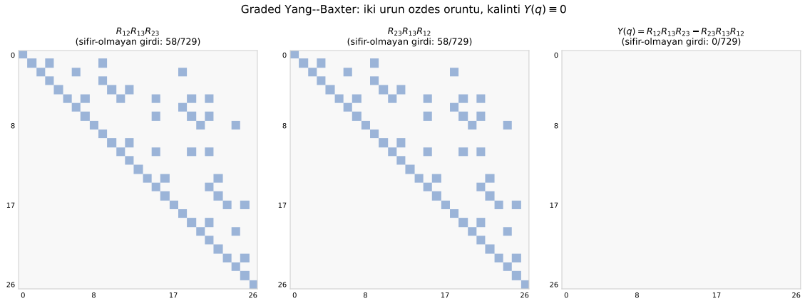
Şekil 9.4 Graded Yang–Baxter denkleminin iki tarafının 27 \times 27 sıfır-olmayan örüntüleri özdeşir; kalıntı Y(q) = R_{12}R_{13}R_{23} - R_{23}R_{13}R_{12} tüm 729 girdide sıfırdır (graded_yang_baxter_residual_GLq21).
