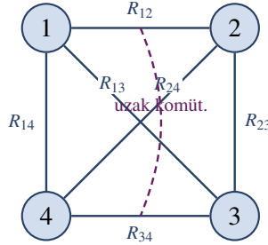
Şekil 9.5 V^{\otimes 4} yerleşimlerinin K_4 grafiği: altı kenar altı R_{ij} , dört üçgen (\{1,2,3\}, \{1,2,4\}, \{1,3,4\}, \{2,3,4\}) dört lokal Yang–Baxter kontrolü, ayrık kenar çifti (12)-(34) ise uzak komütativitedir.
