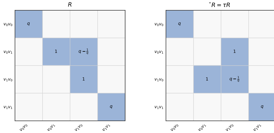
Şekil 8.1 V_1 \otimes V_1 üzerinde Drinfeld R -matrisi ve örgülü \check{R} = \tau R . Renkli hücreler sıfırdan farklı girdileri, içlerindeki ifadeler ise girdinin değerini gösterir (doğrudan R_matrix_V1 / R_check_V1 çıktısı).
