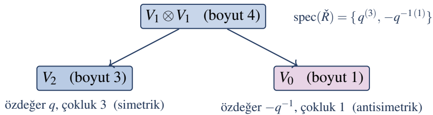
Şekil 8.3 Örgülü \check{R} 'nin spektral ayrışması, V_1 \otimes V_1 = V_2 \oplus V_0 Clebsch–Gordan ayrışımıyla aynıdır. Özdeğer çoklukları doğrudan alt-temsil boyutlarını verir ( R_check_eigenvalues ).
